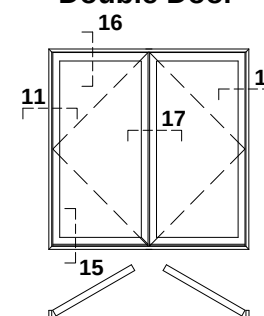
Double Door
