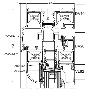
SNEDE 2 COUPE 2
